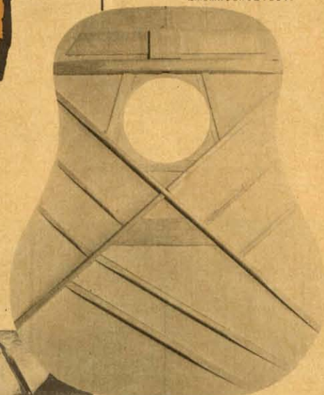
▲Xブレイシング作業(計算された圧力で、熱間をかけた接着法は木と木のなじみを強くします)
