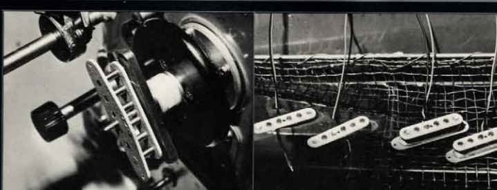
↑コイルのターンとアルニコボールピースが、サウンドの決手。確実にバラフィンで固定されます。ガウスメーターによる磁力検査 →
